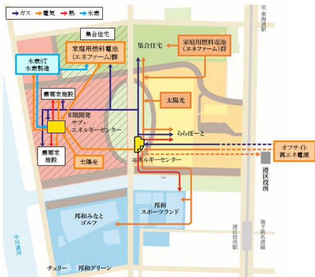
みなとアクルスエネルギー供給図
